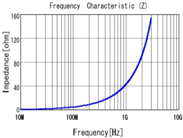
■ LQW2BAS6N8J00 |Z|
