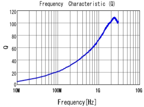
■ LQW2BAS6N8J00 Q
