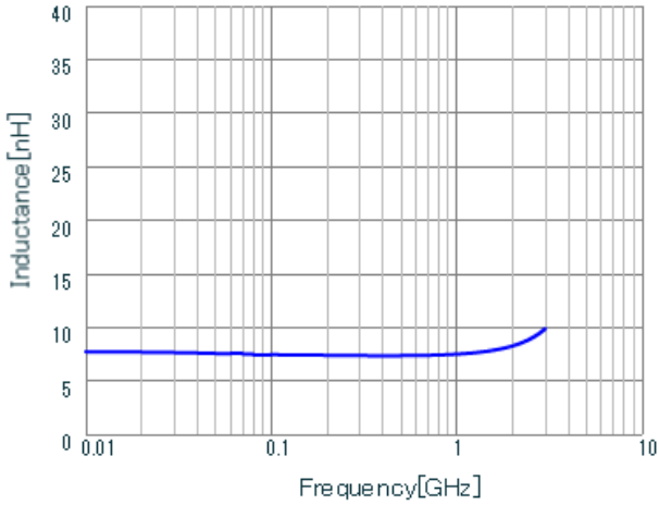
LQW2BAS7N5J00 L.
