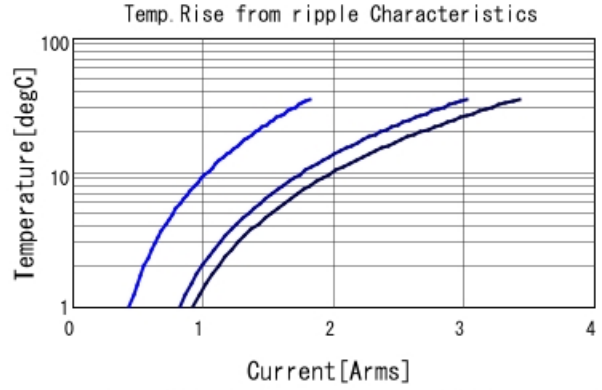
GCM033D70E105ME36 Temp. rise — 100kHz — 500
