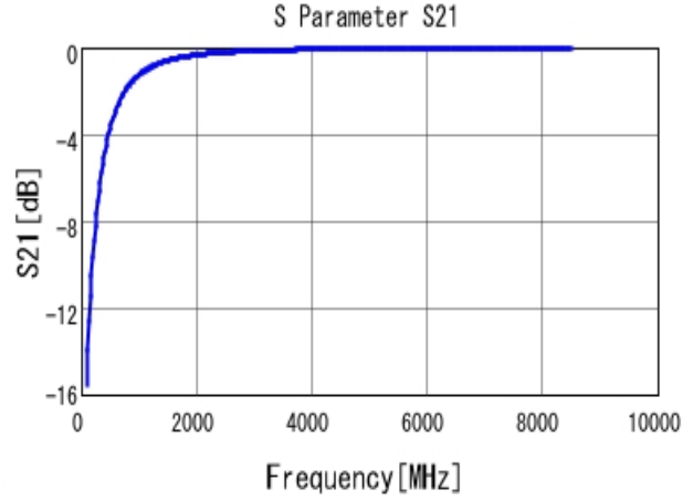
■ GRM0225C1H2R7CA03 S21 DCOV, 25degC
