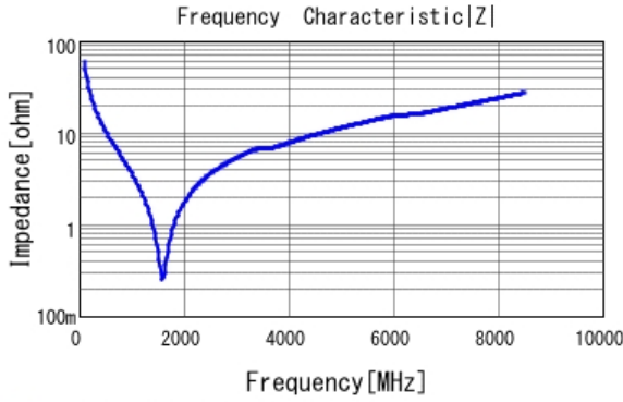
■ GRT1555C2A270JA02 |Z| DC0V, 25degC
