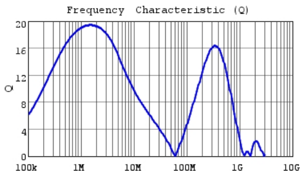
1225AS-H-4R7M Q
