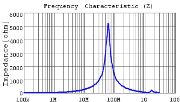
1225AS-H-4R7M |Z|
