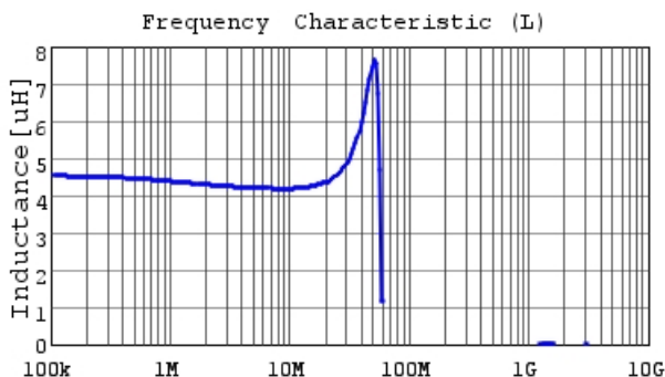
1225AS-H-4R7M L
