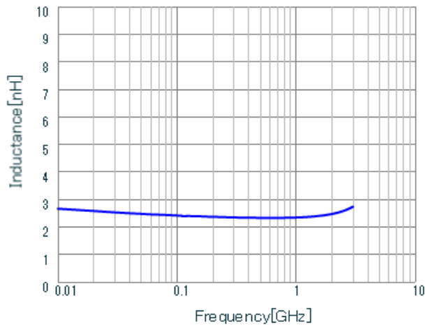
LQG15HN2N4S02 L.
