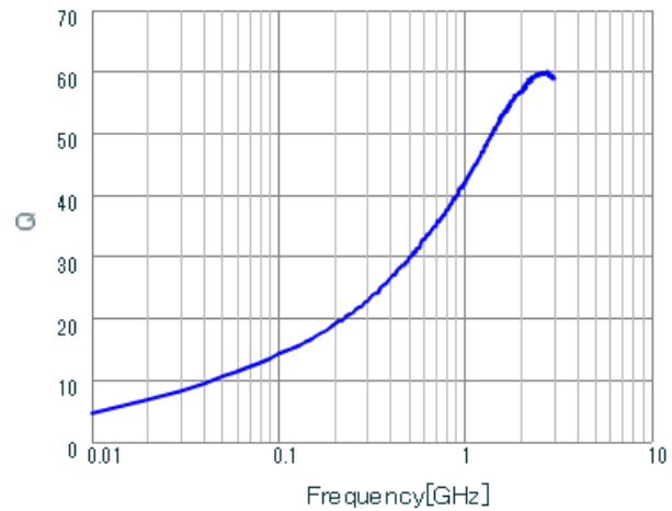
LQG15HN2N4S02 Q.
