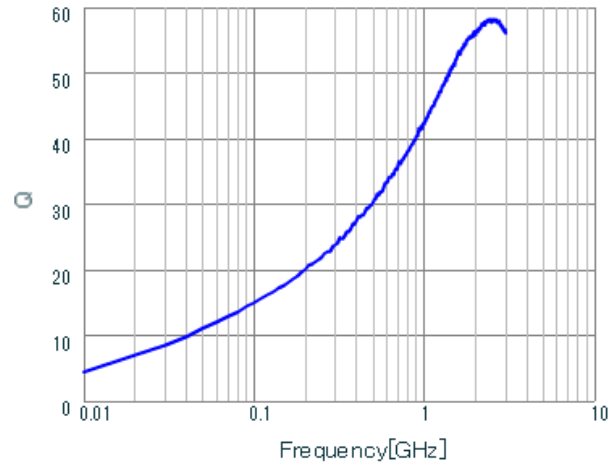
LQG15HN2N7S02 Q.
