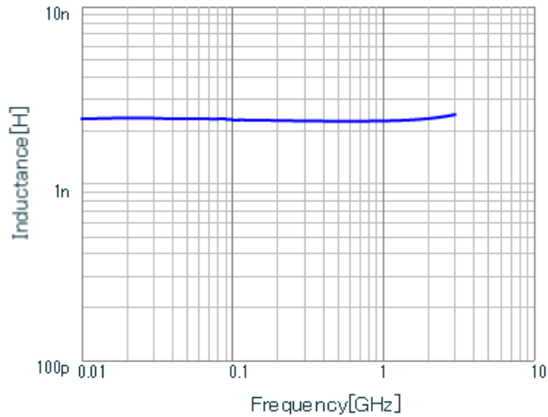
LQG15WH2N3C02 L.
