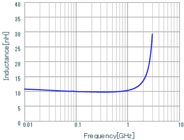
LQG18HN10NJ00 L.
