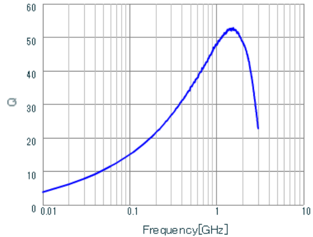
LQG18HN10NJ00 Q.
