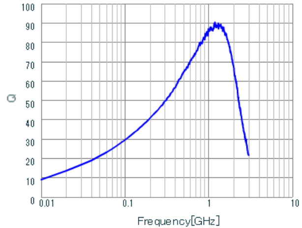
LQW18AN27NG0Z Q.
