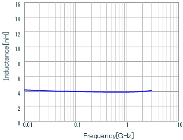
LQW18AN3N9C10 L.
