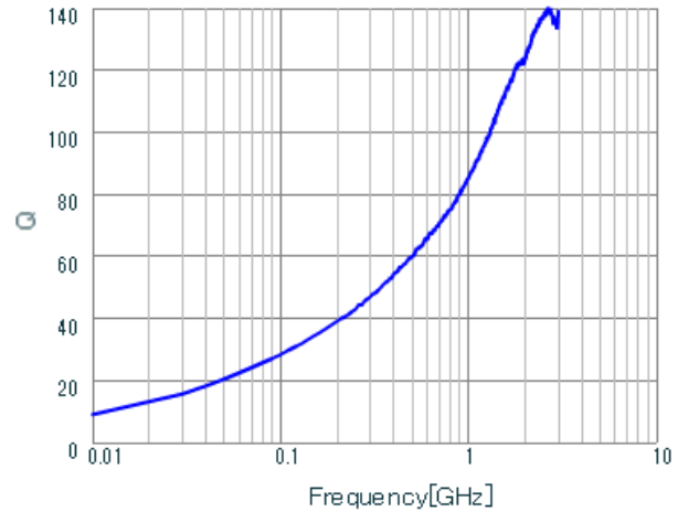
LQW18AN3N9C10 Q.
