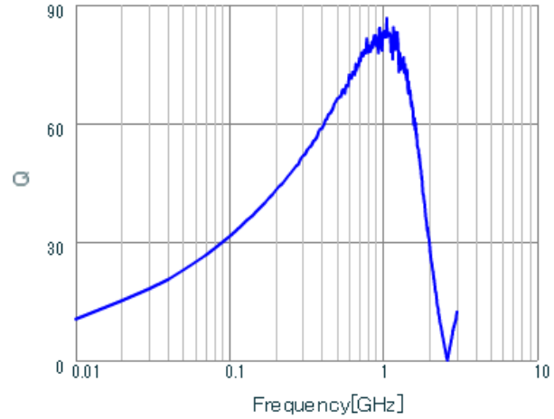
LQW18AN68NG0Z Q.
