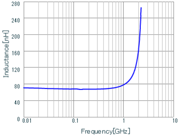
LQW18AN68NG0Z L.
