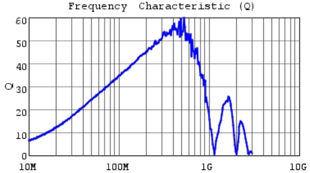
LQW18ANR33G80 Q
