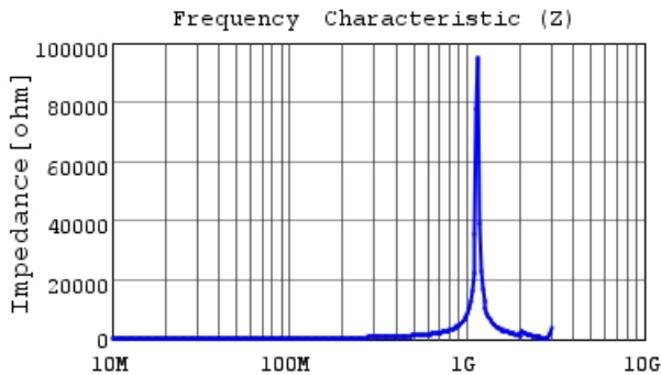
LQW18ANR33G80 |Z|
