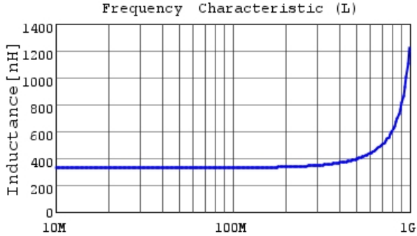
LQW18ANR33G80 L
