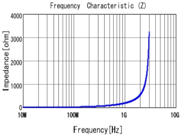
■ LQW2BAS27NG00 |Z|
