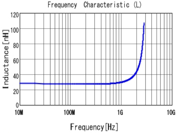
■ LQW2BAS27NG00 L
