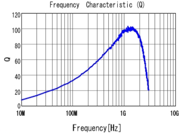
■ LQW2BAS27NG00 Q
