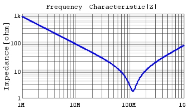
DE1B3RA221KA4BQ01F |Z| DCOV, 20degC
