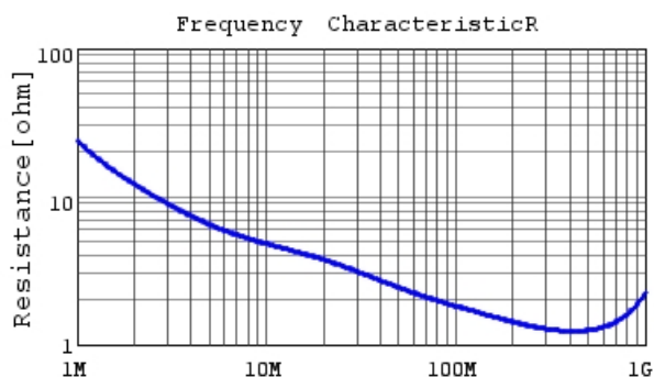
DE1B3RA221KA4BQ01F R DCOV, 20degC
