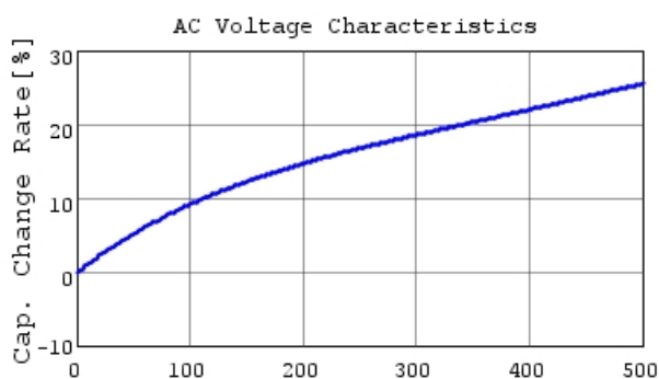
DE1B3RA221KA4BQ01F C-AC Voltage capchange, 1
