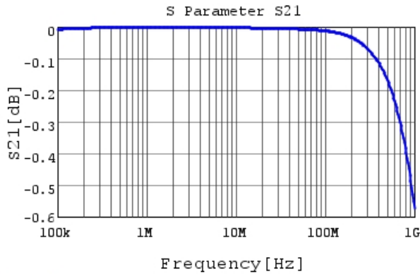
RHEL81H474K2M1H03A S21 DCOV, 25degC
