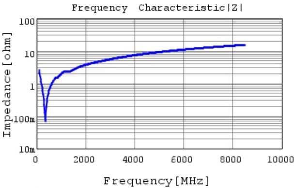
GCM1555C1H561FA16 |Z| DCOV,25degC
