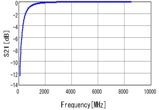
S Parameter S21
