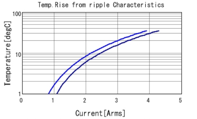
■ LLC152D70G105ME01 Temp. rise — 500kHz — 1MHz
