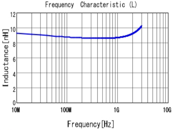
■ LQW15AN8N8G00 L
