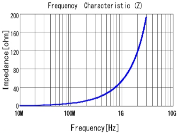
■ LQW15AN8N8G00 |Z|
