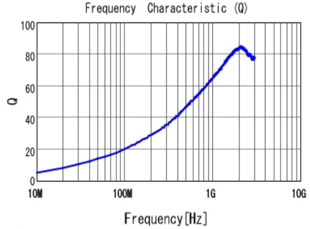
■ LQW15AN8N8G00 Q
