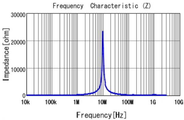
#B953AS-330M=P3 |Z|
