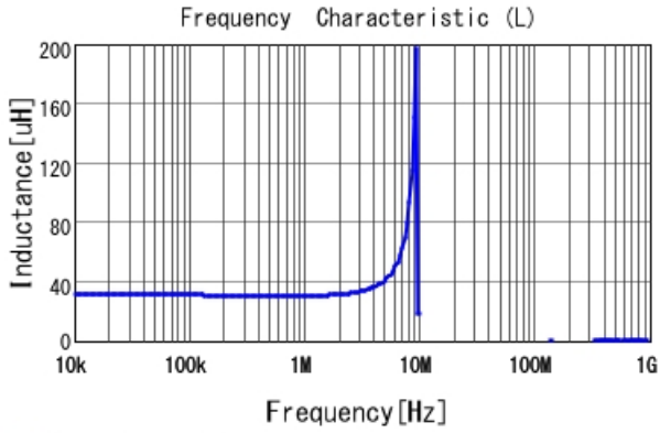
#B953AS-330M=P3 L
