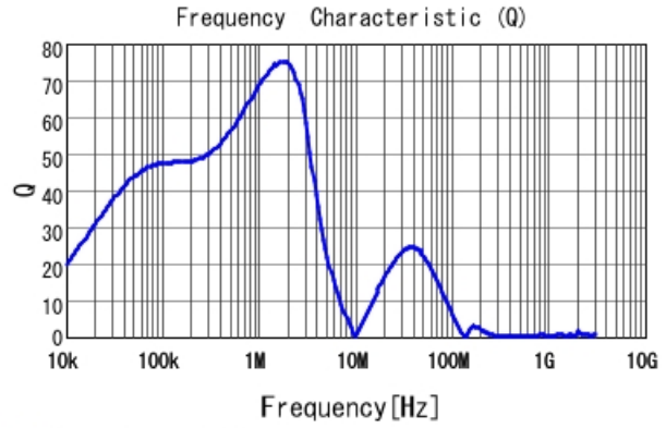
#B953AS-330M=P3 Q
