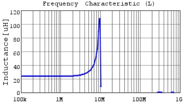
DFEH7030D-220M L
