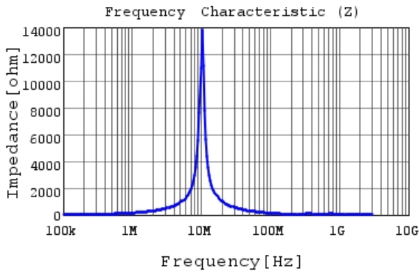
DFEH7030D-220M |Z|
