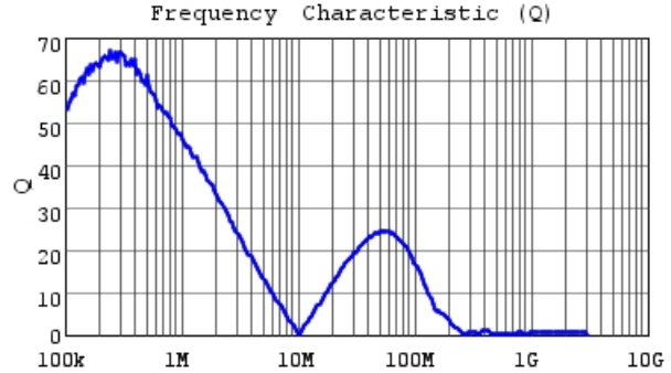
DFEH7030D-220M Q
