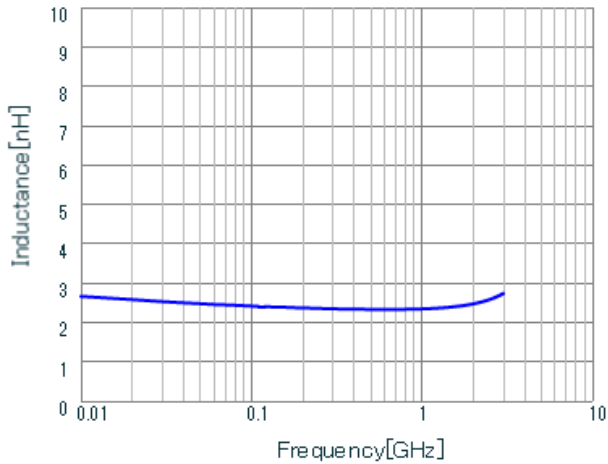
LQG15HN2N4S02 L.
