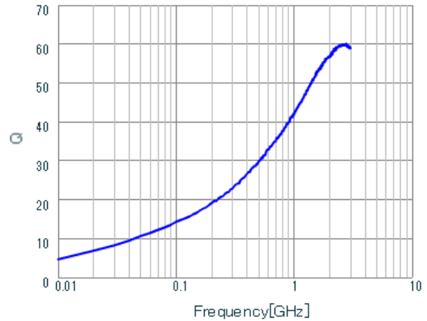
LQG15HN2N4S02 Q.
