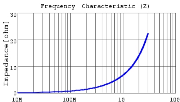
LQG15HZ1N1B02 |Z|
