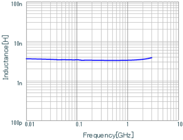
LQG15WZ3N4S02 L.
