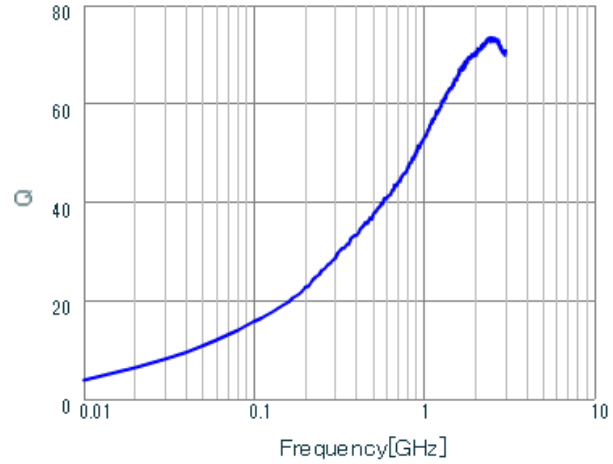
LQG15WZ3N4S02 Q.
