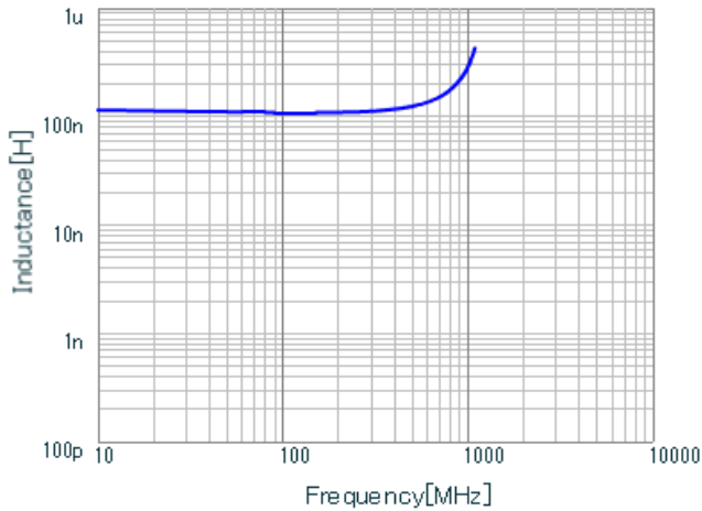
LQG15WZR11J02 L.
