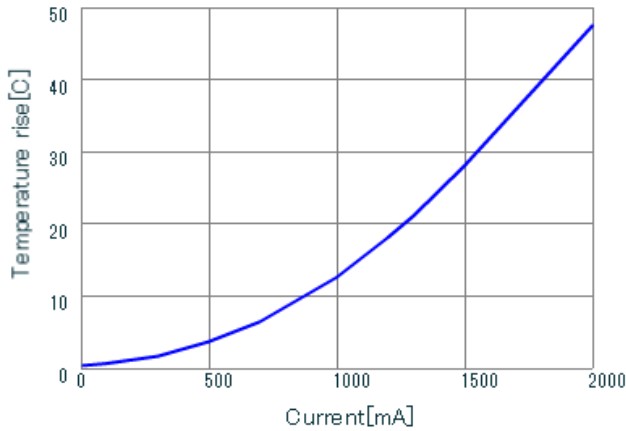
LQM31PN1R0M00 DT_Current
