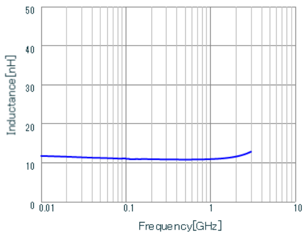
LQW15AN11NG00 L.
