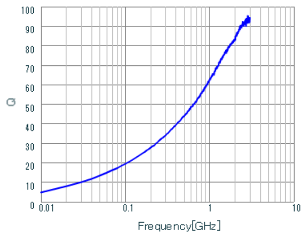
LQW15AN11NG00 Q.
