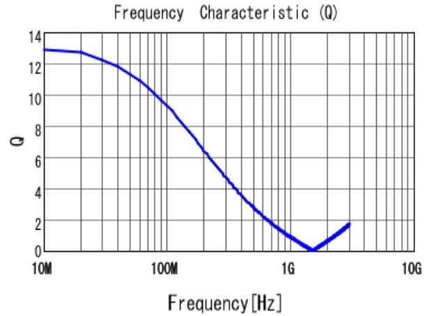
■ LQW15CAR22K00 Q
