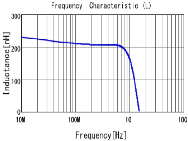
■ LQW15CAR22K00 L
