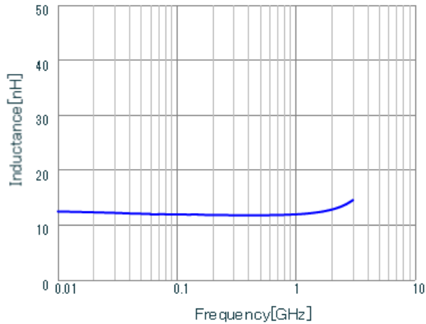
LQW18AN12NG0Z L.
