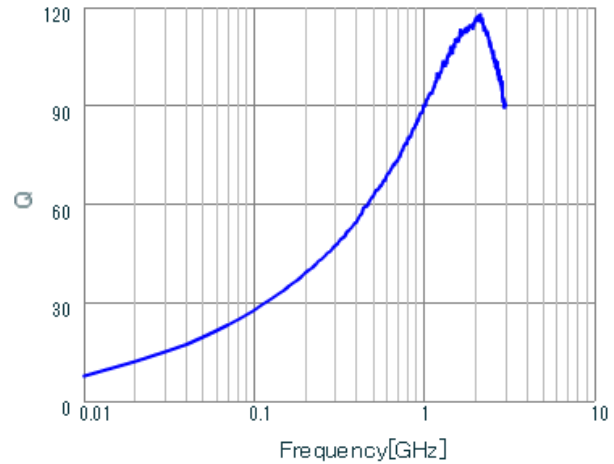
LQW18AN12NG0Z Q.
