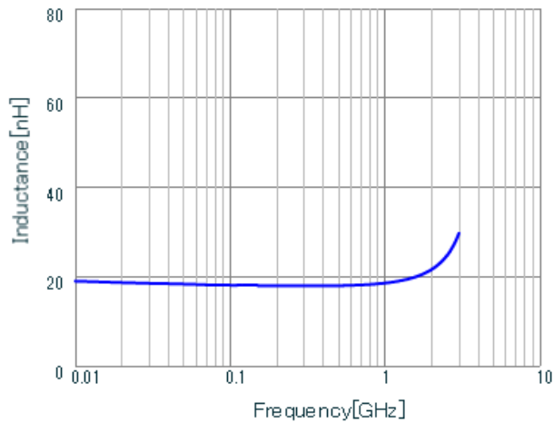
LQW18AN18NG00 L.
