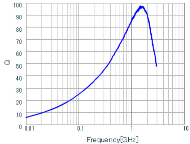
LQW18AN18NG00 Q.
