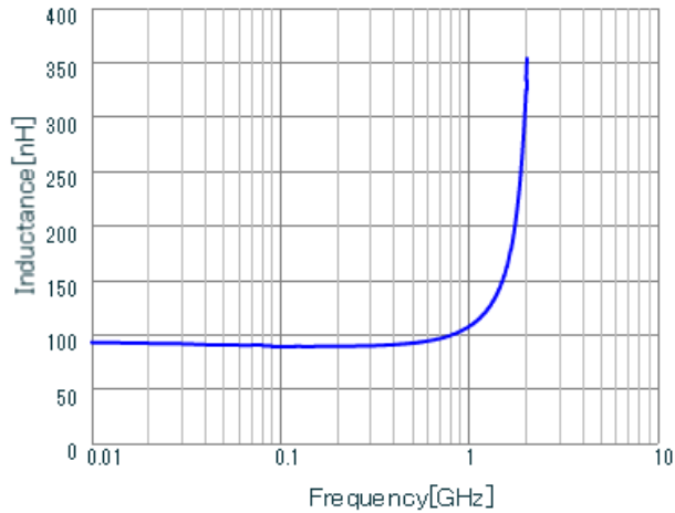
LQW18AN91NG0Z L.
