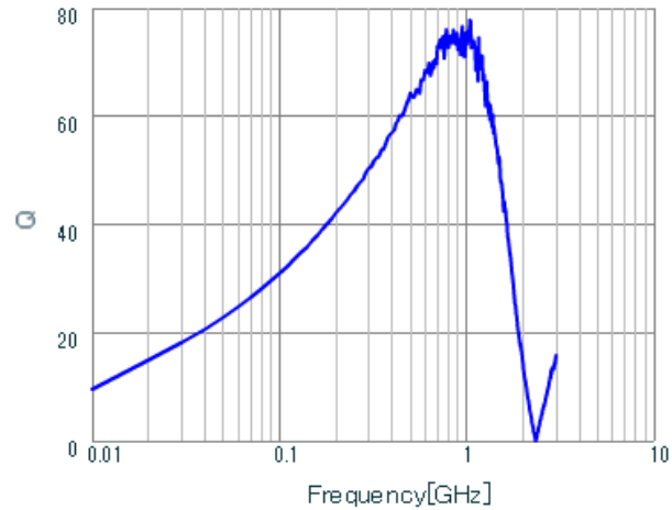
LQW18AN91NG0Z Q.
