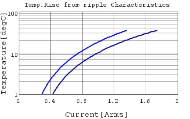
GRM155R60J224KE01 Temp.rise 500kHz
