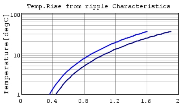
GRM21BR71H154KA01 Temp.rise — 500kHz —
