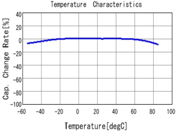
■ GRM035R60J475ME15 C-Temp. capchange, DCO. 0V, ACO. 1V rm
