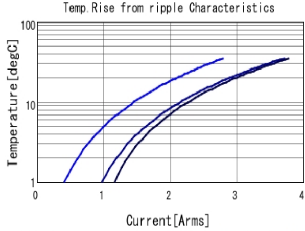
GRM035R60J475ME15 Temp. rise ■ 100kHz ■ 500kHz ■ 1MHz
