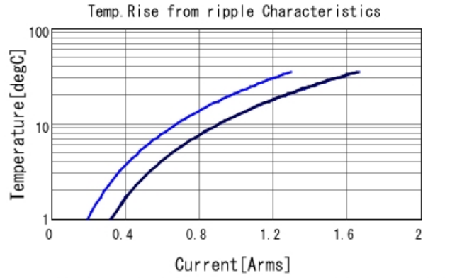
GRM188R72A104KA35 Temp. rise — 400kHz — 800
