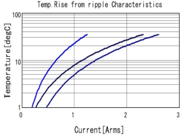
GRM21BR71H474KA88 Temp. rise ■ 100kHz ■ 500kHz ■ 1MHz
