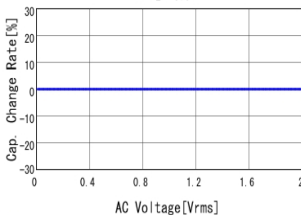
AC電圧特性
