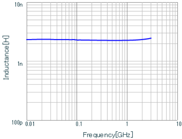
LQG15WH2N3C02 L.
