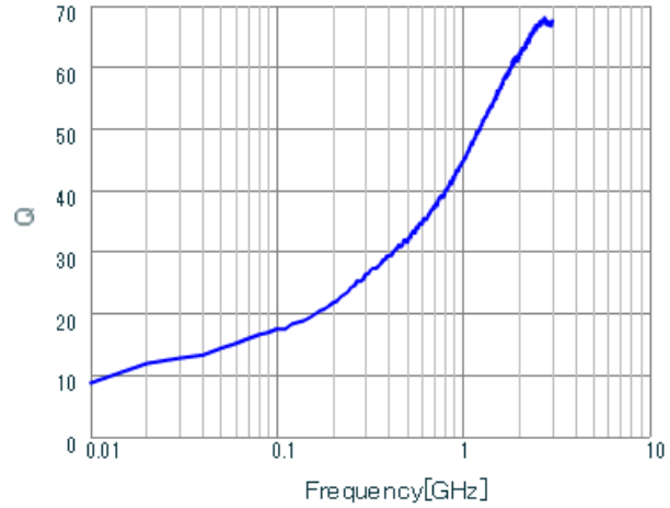
LQG15WH2N6C02 Q.
