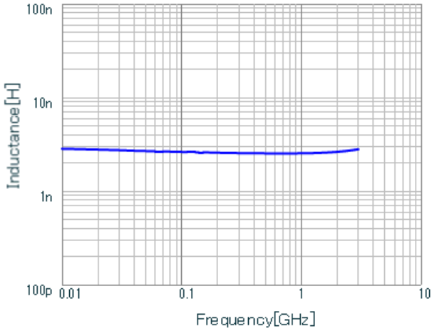
LQG15WH2N6C02 L.
