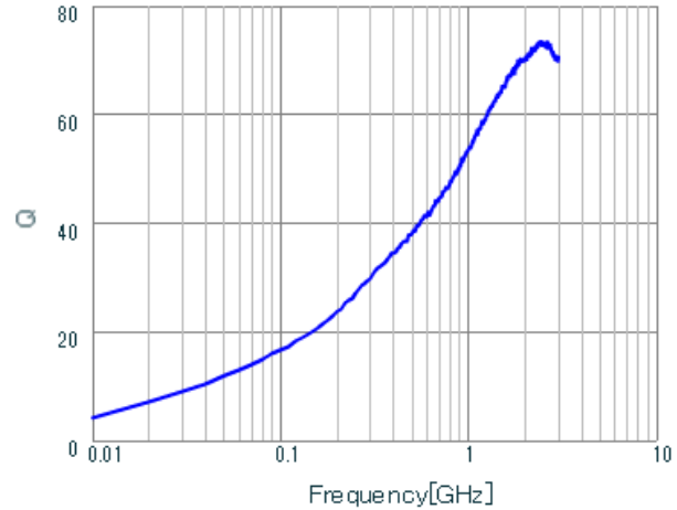
LQG15WH3N7C02 Q.
