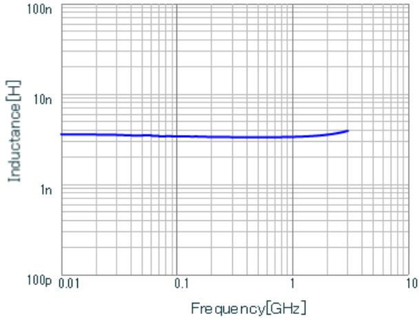
LQG15WH3N7C02 L.
