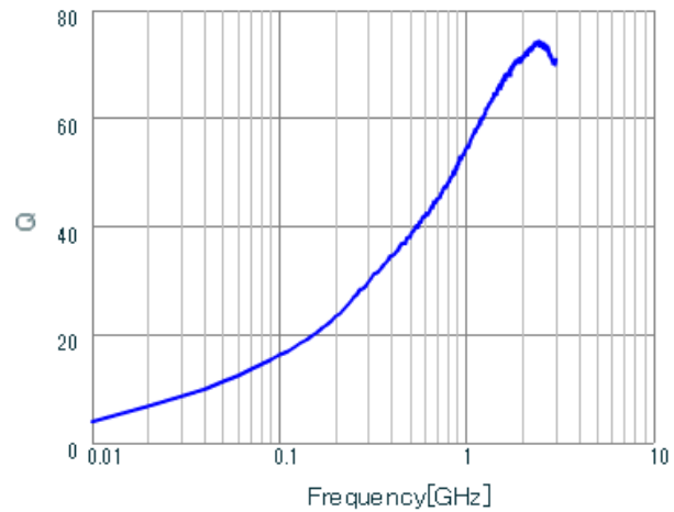
LQG15WH3N8C02 Q.
