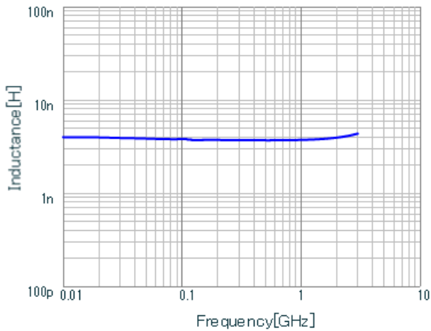
LQG15WH3N8C02 L.
