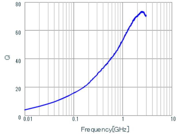
LQG15WZ3N4S02 Q.
