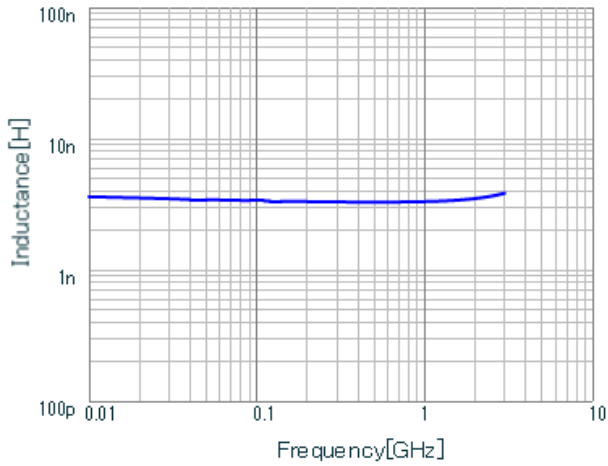
LQG15WZ3N4S02 L.
