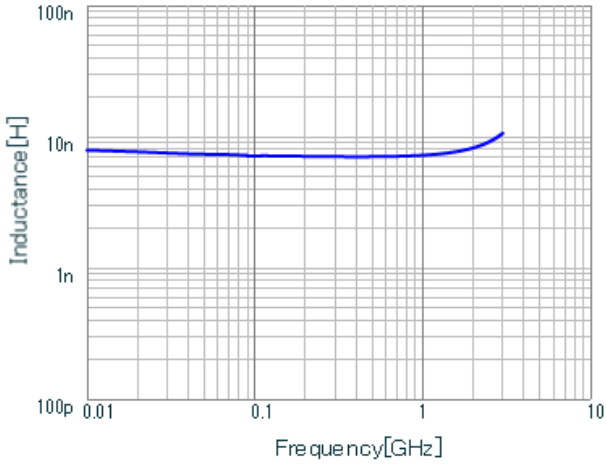
LQG15WZ7N3G02 L.
