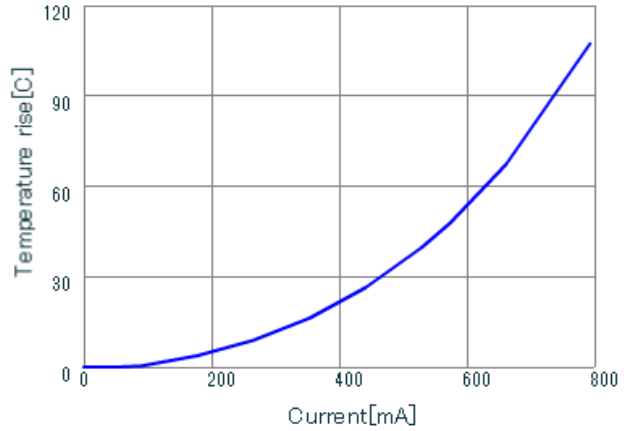
LQH3NPN470MMR DT_Current
