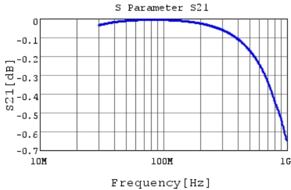
RHE5G1H561J0M1H03A S21 DCOV, 25degC
