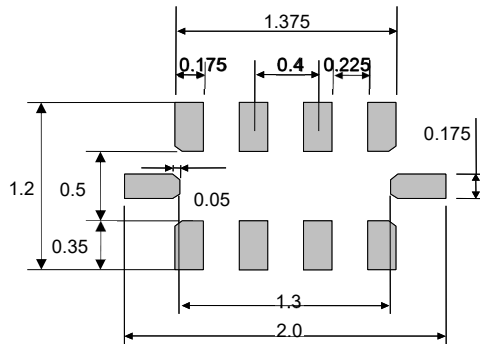
クリームはんだ標準塗布パターン
