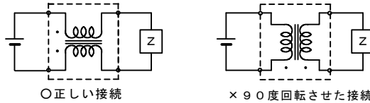
○正しい接続
