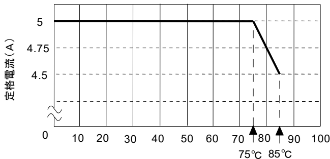
DLW5BSM191の使用温度デレティンク
